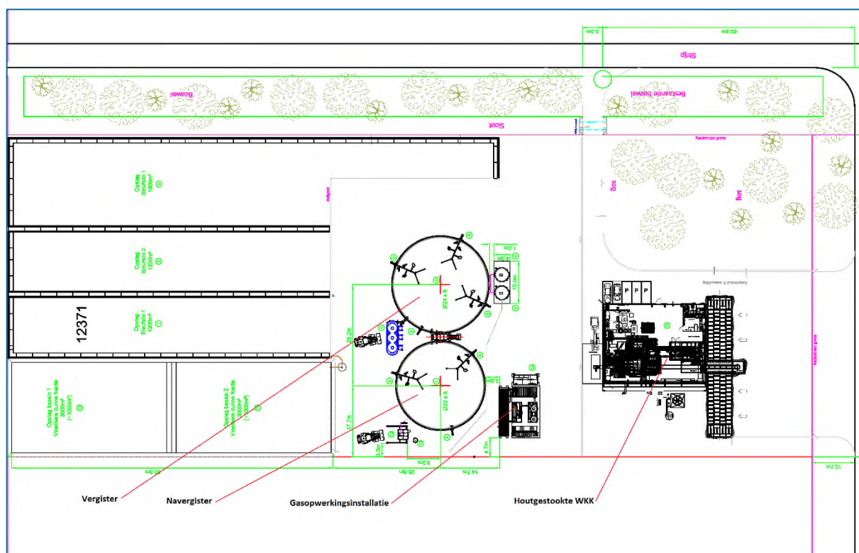
Figuur 3.4 Een aantal voor de QRA mogelijk relevante onderdelen van de bigasinrichting
