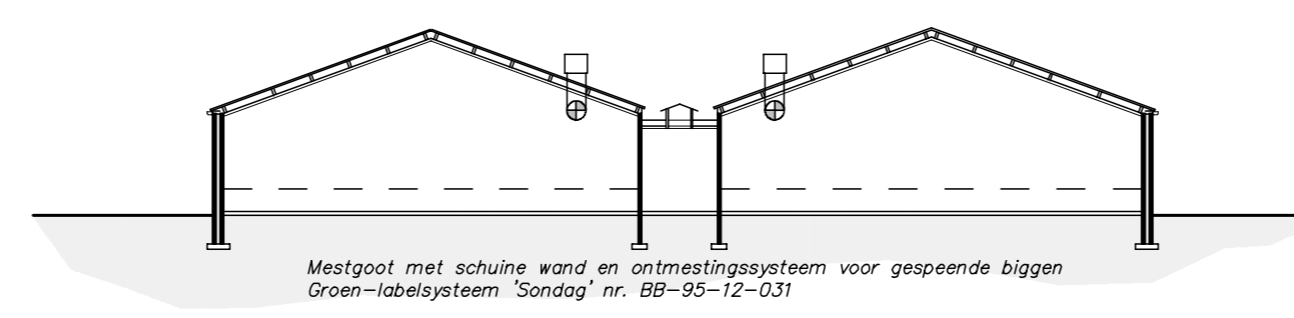
DOORSNEDE E - E
