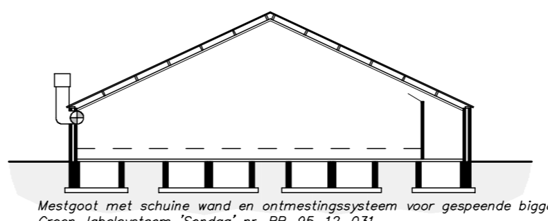
DOORSNEDE D - D
