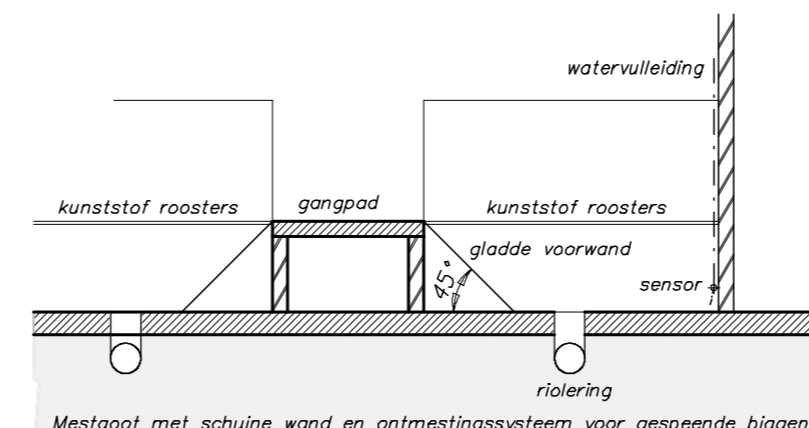
PUTPRINCIPE SONDAG 1 : 50
