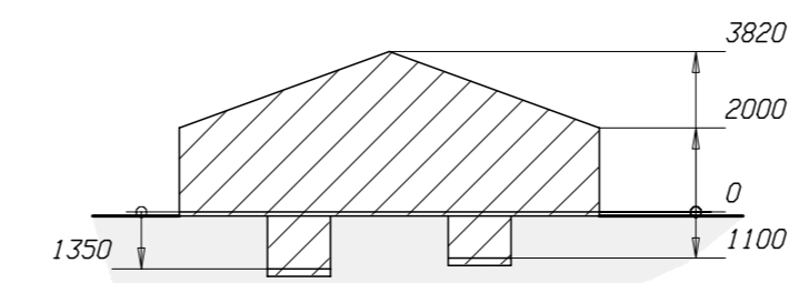
DOORSNEDE B - B
