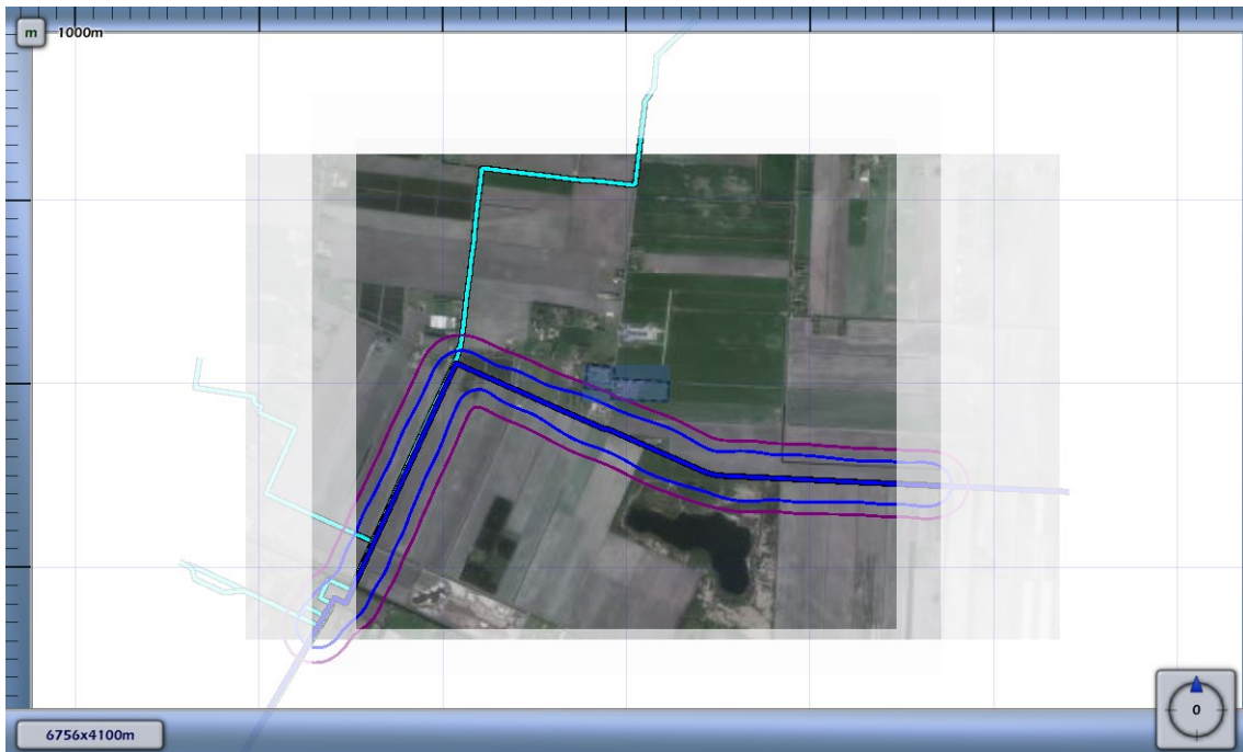
3.2 Figuur 3.4 Plaatsgebonden risico voor N-522-62 van N.V. Nederlandse Gasunie
