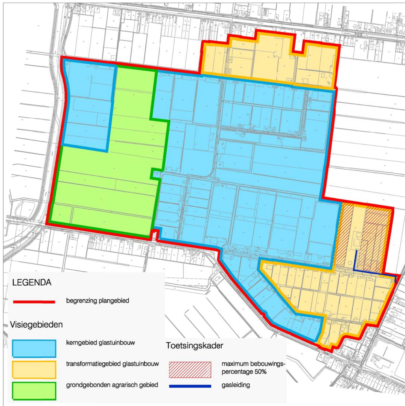
Figuur 2 Structuurvisiekaart
