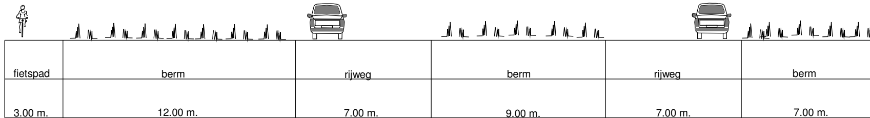
Dwarsprofiel Rondweg Emmen-Emmerhout
