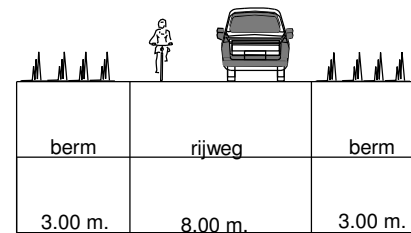
Dwarsprofiel Laan van de Marel Emmen-Emmerhout
