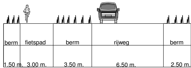
Dwarsprofiel Houtweg Emmen-Emmerhout
