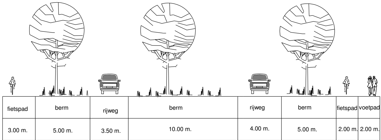
Dwarsprofiel Statenweg Emmen-Angelslo
