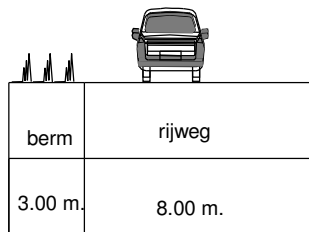
Dwarsprofiel Boerschapslaan Emmen-Angelslo
